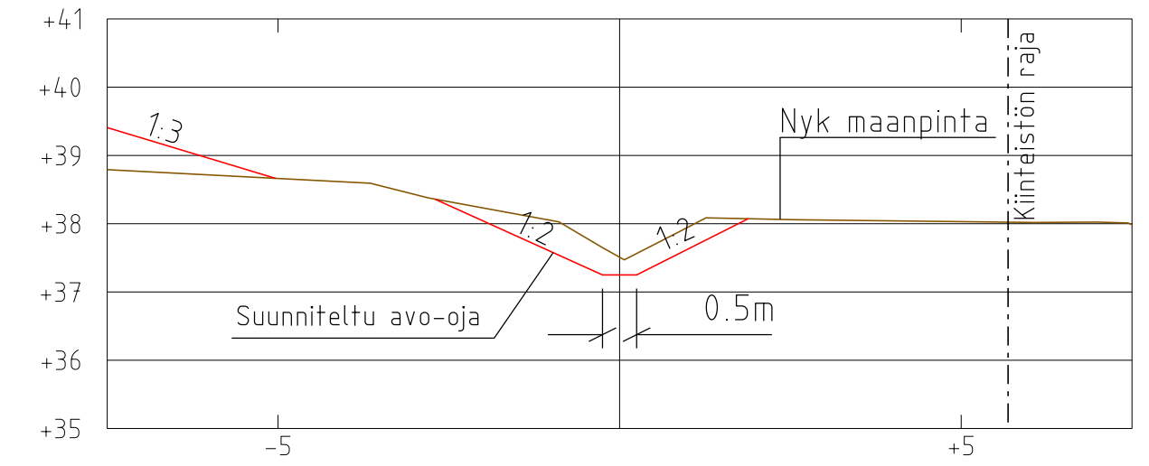
TYYPPIPOIKKILEIKKAUS 1:100 PAALU 100
